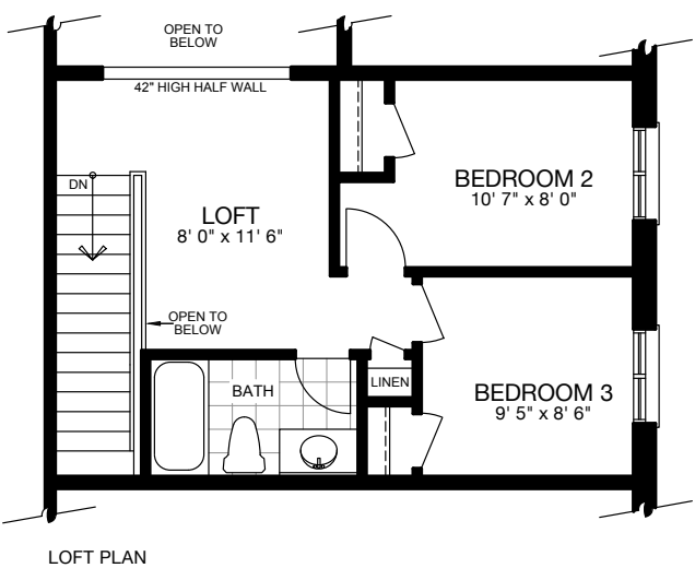
LOFT PLAN
